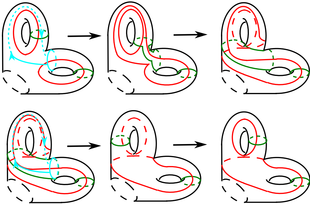
FIGURE 3. D_\omega^{-1} D_\theta^{-1} D'_\omega D_\theta
